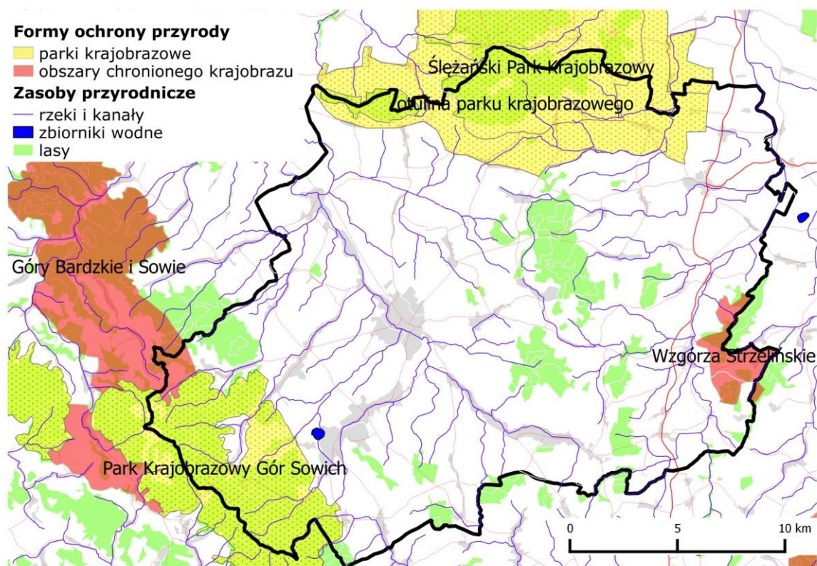
Rys. 3 Najważniejsze obszary chronione w powiecie dzierżoniowskim
