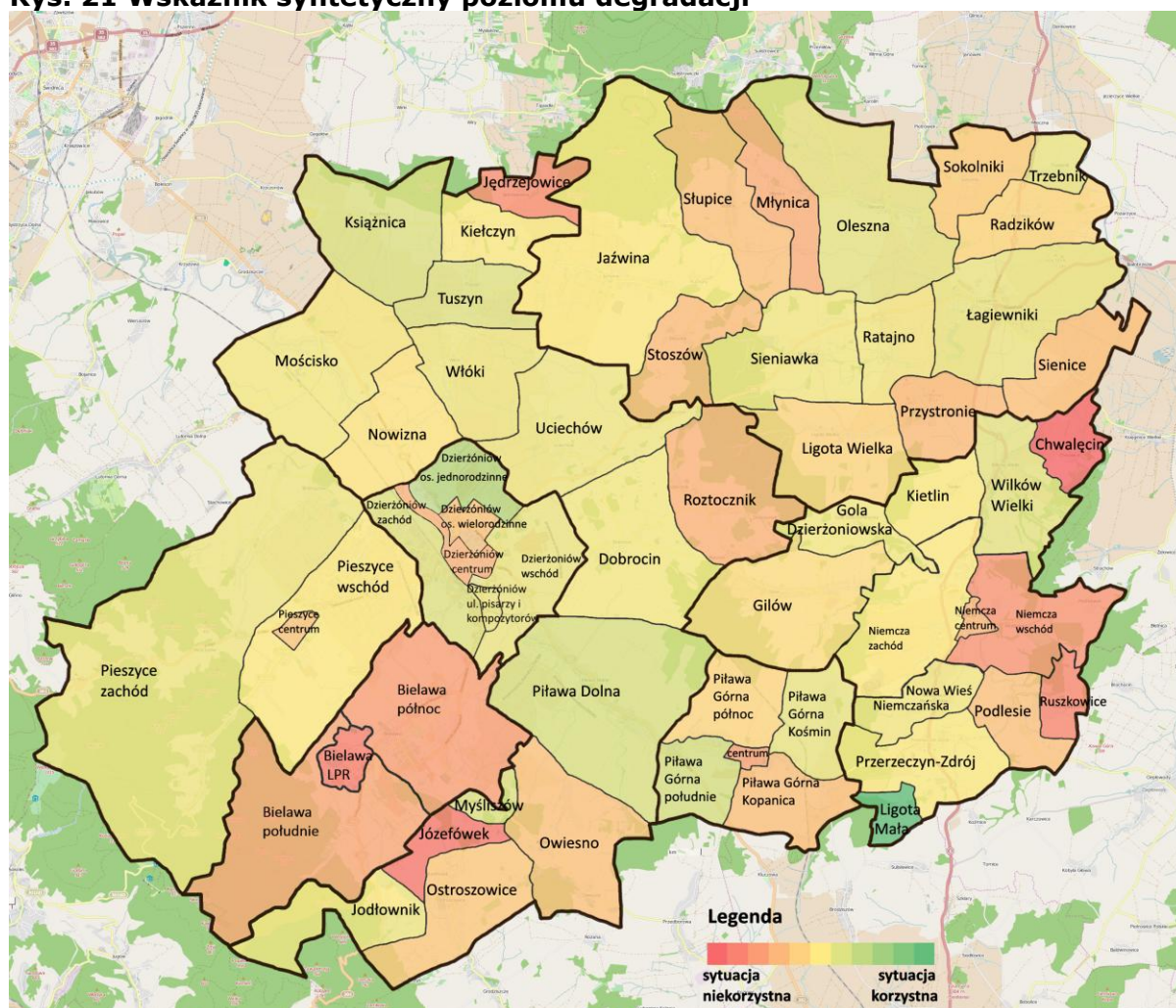
Rys. 21 Wskaźnik syntetyczny poziomu degradacji
